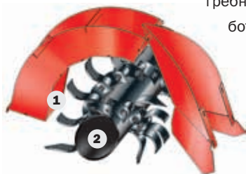
Отличный результат: большие размеры роторного вала (2) убеждают своим тихим ходом и стабильностью. Противорежущая пластина (1) заботится о чистом срезе.
