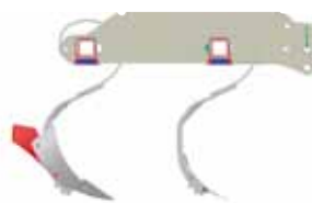
Подпружиненный окучивающий корпус 5 с подпружиненными плоскими лапами (жесткий монтаж к раме) 5
